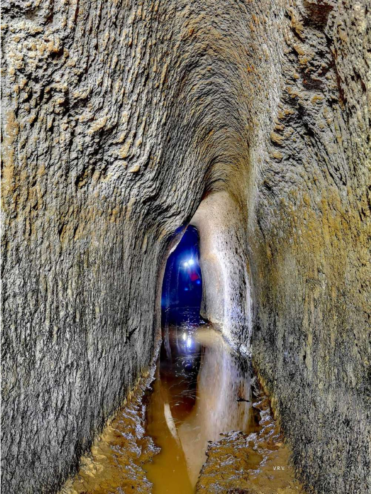
FIG.15 galleria di drenaggio delle acque superficiali area VT16
